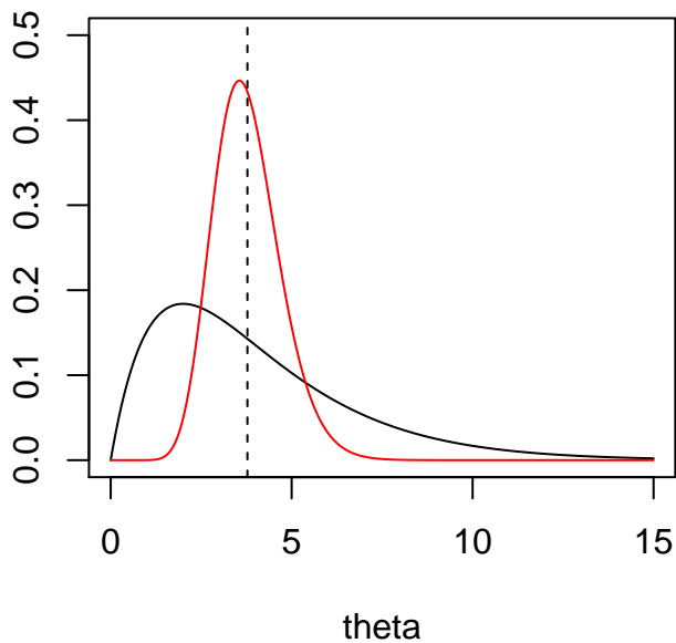
theta~Gamma(2,2)
