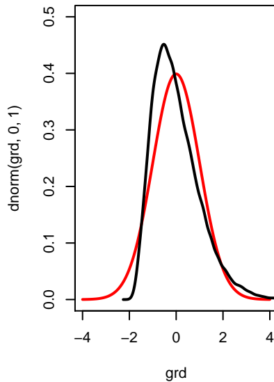
n=4
