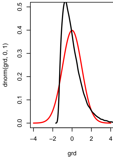
n=2
