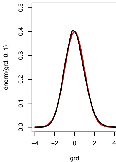
n=100
