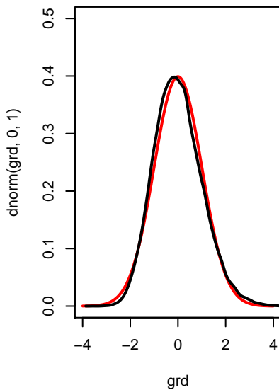
n=30
