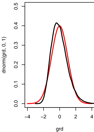
n=10
